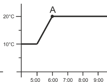
Teplota miestnosti - zapnutá funkcia OPTIMUM START:
