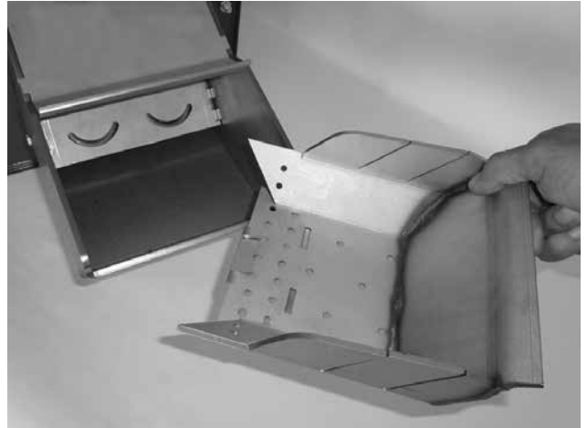
Obr. 2 - vyjímatelná spalovací komůrka - nutno pravidelně čistit
