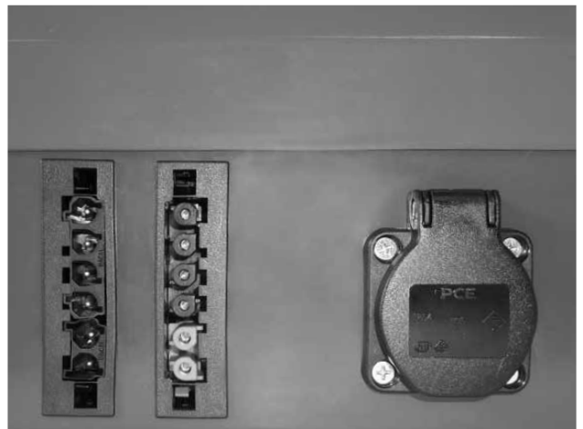
Obr. 12 - hořák - dva 6-pinové konektory, levý silový, pravý pro čidla a zasuvka pro dopravník
